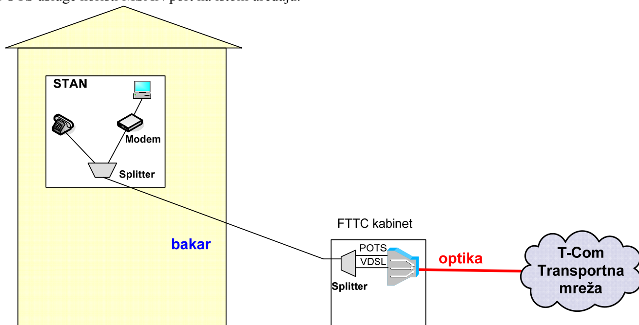
30. Način realizacije FTTC koncepta u pristupnoj mreži
