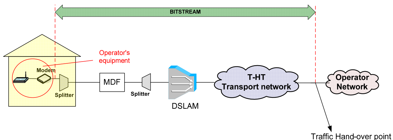
Slika 31. Koncept posebnog virtualnog kanala za Podatkovnu uslugu
