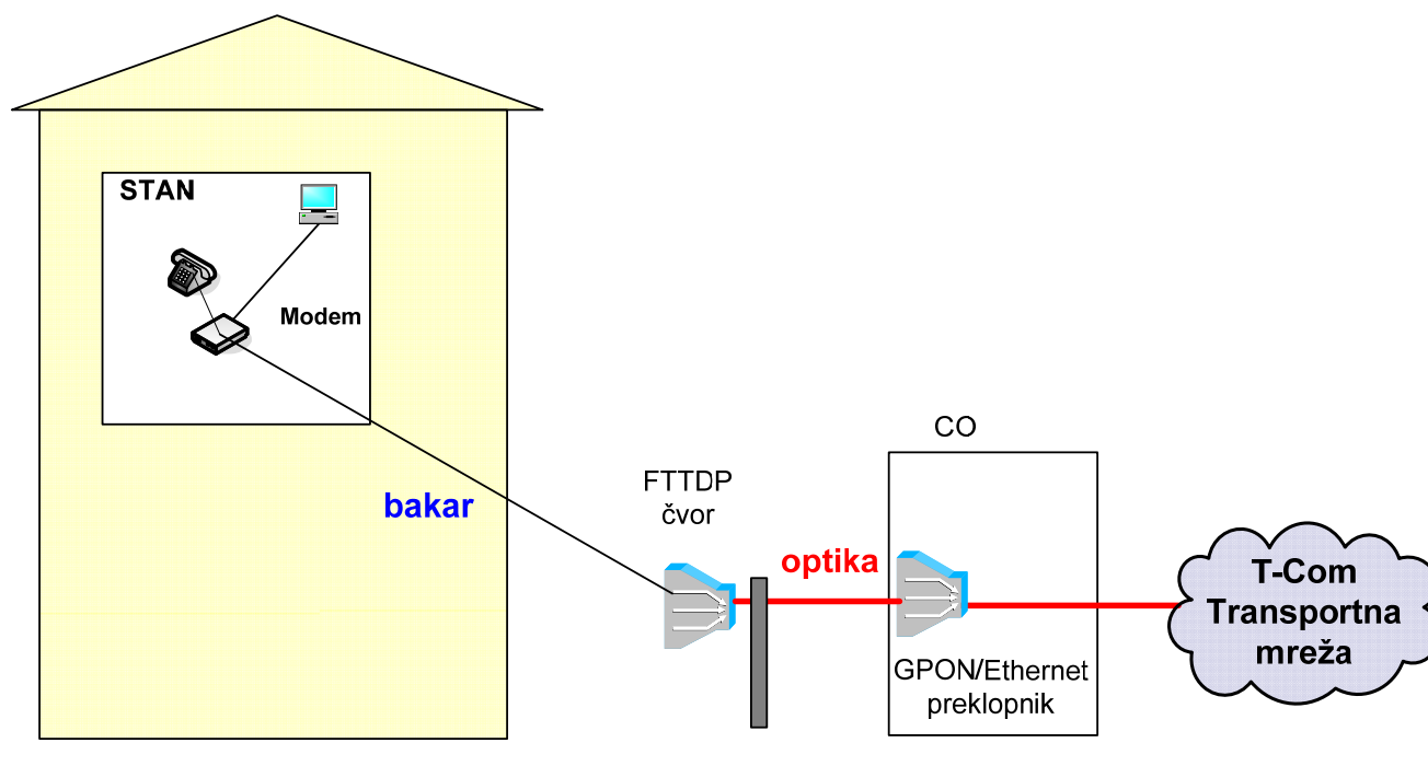
Slika 35. Način realizacije FTTDP koncepta u pristupnoj mreži
