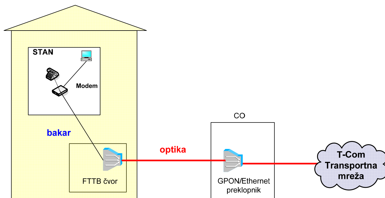
Slika 34. Način realizacije FTTB koncepta u pristupnoj mreži
